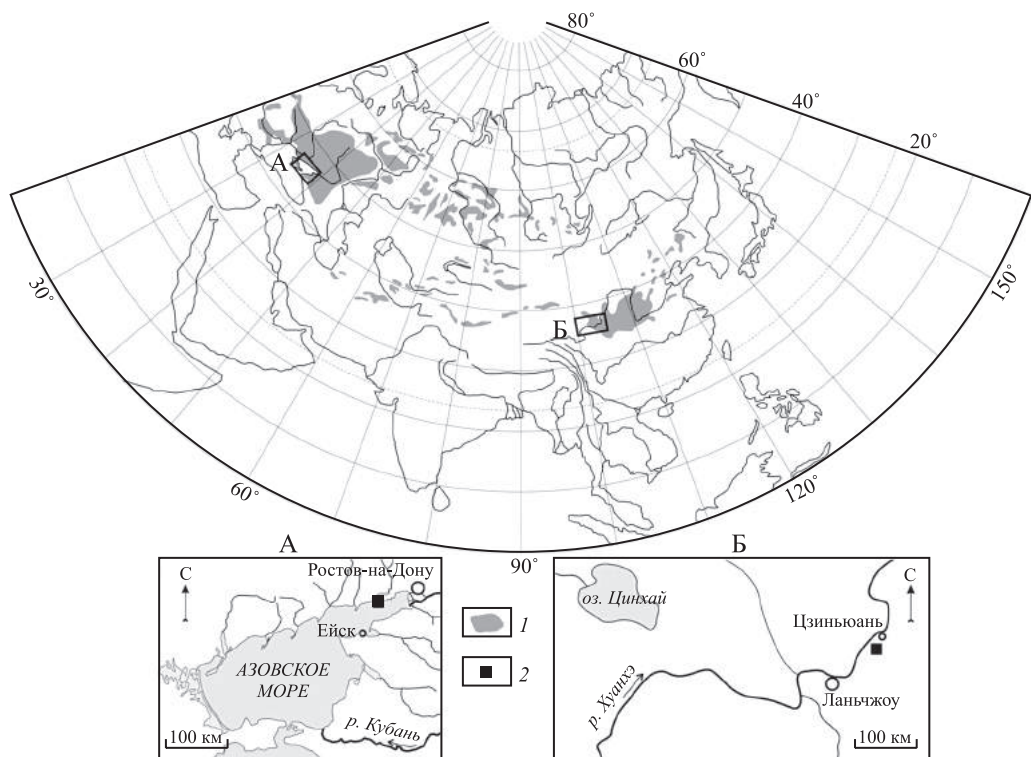
Рис. 1. Распространение типичных лёссов в Евразии (1) по [1, 2] и положение объектов исследования (2): А — Беглиця-2, Б — Цаюсянь
