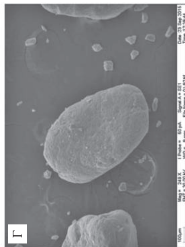
Рис. 3. Морфологические особенности песчаных кварцевых зёрен Разрез Веглица-2 : А – хорошо окатанное зёрно из позднеледниковой лёссово-песчаной толщи со следами криогенной обработки, В – кварцевое зёрно из лёссово-песчаной толщи с бугристо-ямчатой поверхностью и со следами химического выветривания. Разрез Цао-сянь : Г – хорошо окатанное зёрно из лёссово-песчаной толщи, Д – зёрно из лёссово-песчаной толщи с бугристо-ямчатой поверхностью, Е – зёрно из погребённой почвы с бугристо-ямчатой поверхностью
